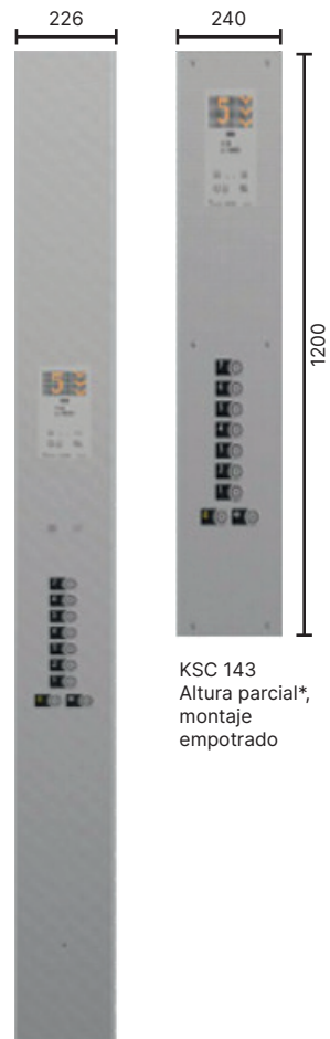
KSC 143 Altura total* Montaje empotrado
