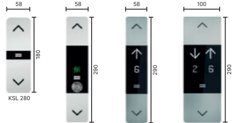
KSL 280 KSL 284 KSL 286 simplex KSL 286 duplex KLX02 Acabados: ST4 Silver, acero inoxidable cepillado y CB Carbon Black, acero inoxidable pulido (antihuellas)
