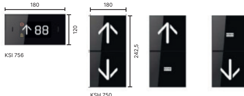
KSI 756 KSH 750 Acabados: ST4 Silver, acero inoxidable cepillado y CB Carbon Black, acero inoxidable pulido (antihuellas)
